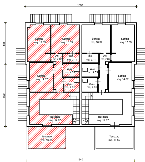
PRIMO PIANO
