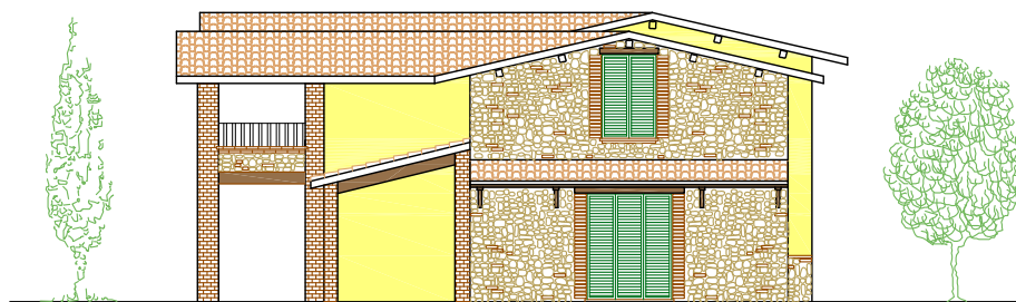
PROSPETTO SUD
