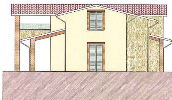
PROSPETTO NORD
